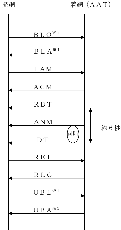
図5. 3-1 課金レート無し，強制切断無し，AAT接続の信号シーケンス
